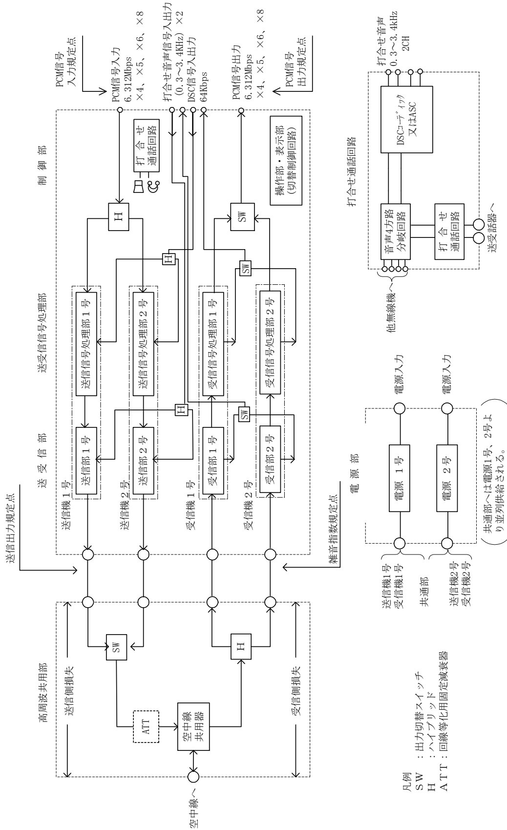
付図1 7. 5GHz帯16QAM多重無線装置系統図(単一受信方式)
