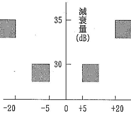
周波数 (MHz) 等価送信ろ波器特性
