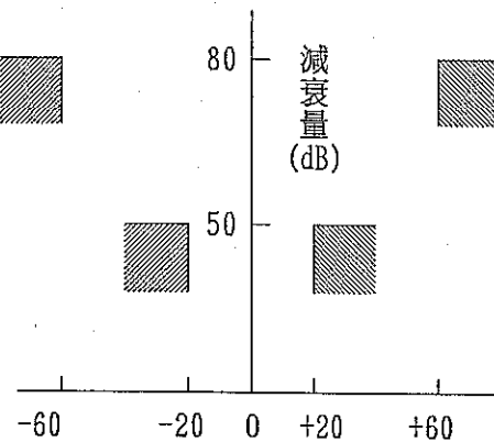
周波数 (MHz) 等価受信ろ波器特性
