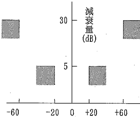
周波数 (MHz) 送信ろ波器特性
