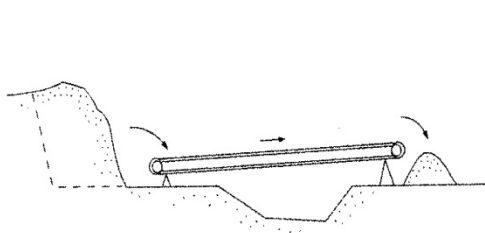
図3.1 水平据付
