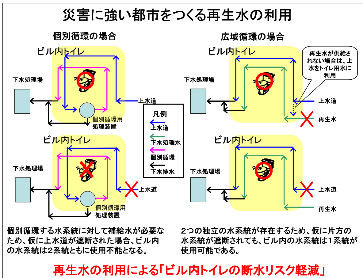
図3 ビル内の雑用水利用形態によるトイレの機能停止リスク
