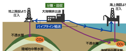
二酸化炭素の回収・貯留のイメージ
