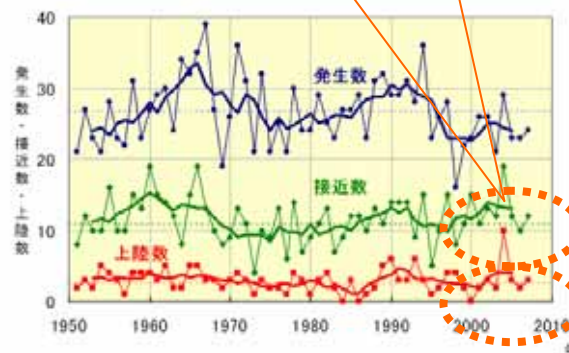
太い実線はそれぞれの5年移動平均。 細い波線はそれぞれの年平均値(1971~2000年の平均値)
