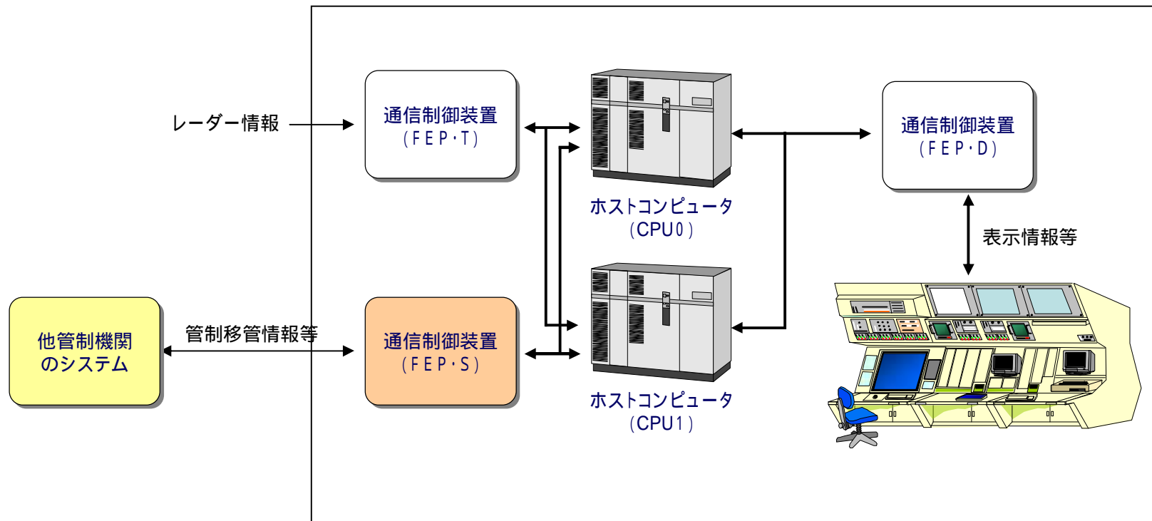
航空路レーダー情報処理システム(RDP)構成概略図
