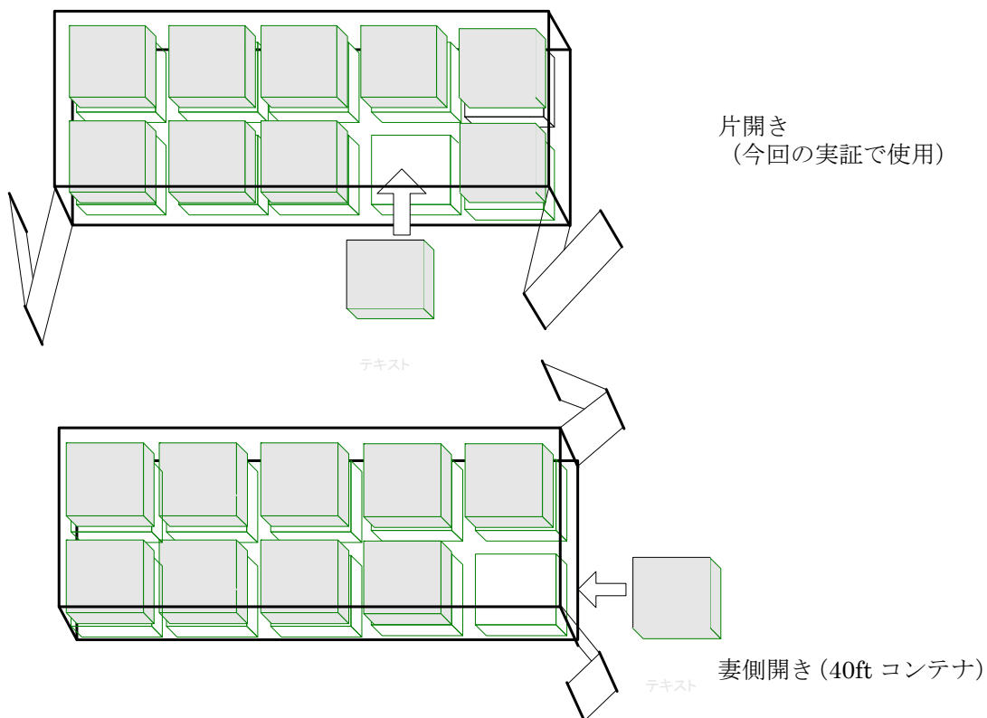
図 2-7 コンテナの積込パターン
