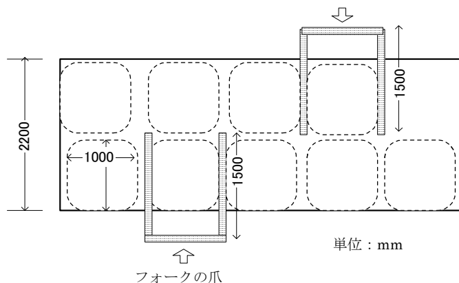
図 2-6 フォークの爪とコンテナの 積込イメージ
