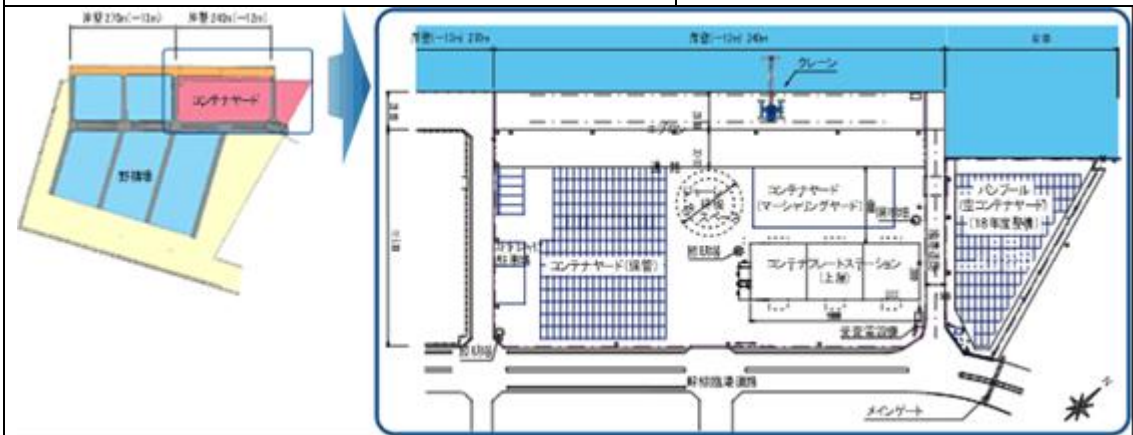
コンテナヤード平面
