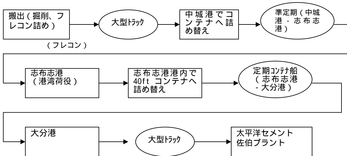
図3 - 6 1 物流フロー（ケース4）
