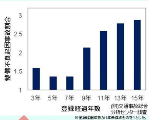
登録経過年別整備不良起因事故割合
