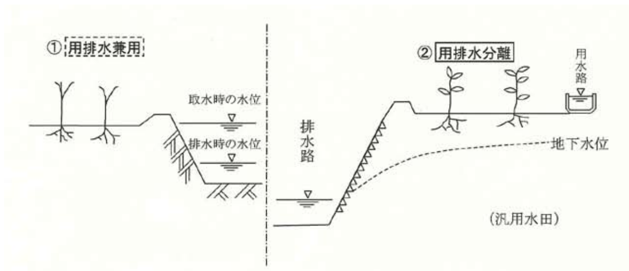
参考 2-4-2 用排水の分離による汎用田化
