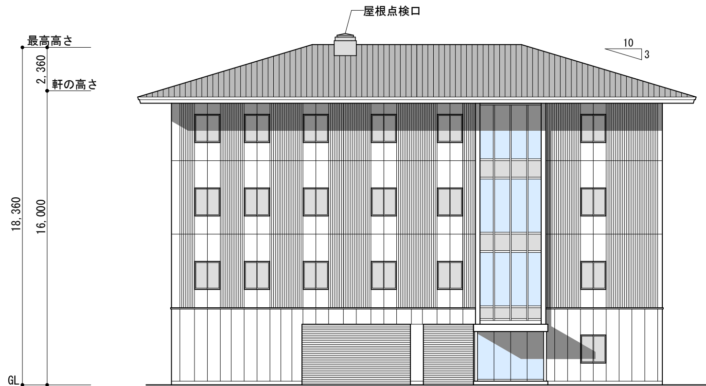
北側 立面図 1/200
