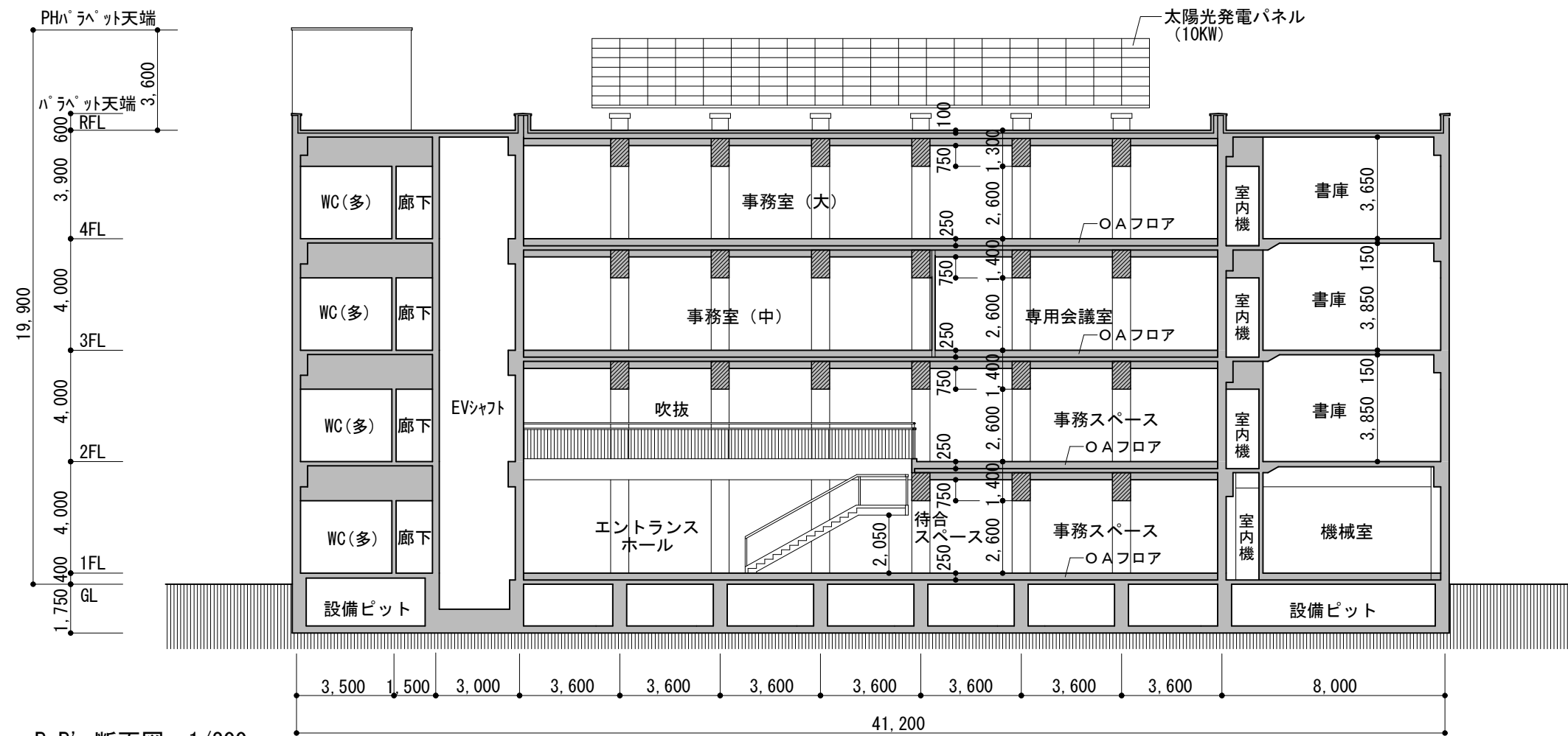
B-B' 断面図 1/200
