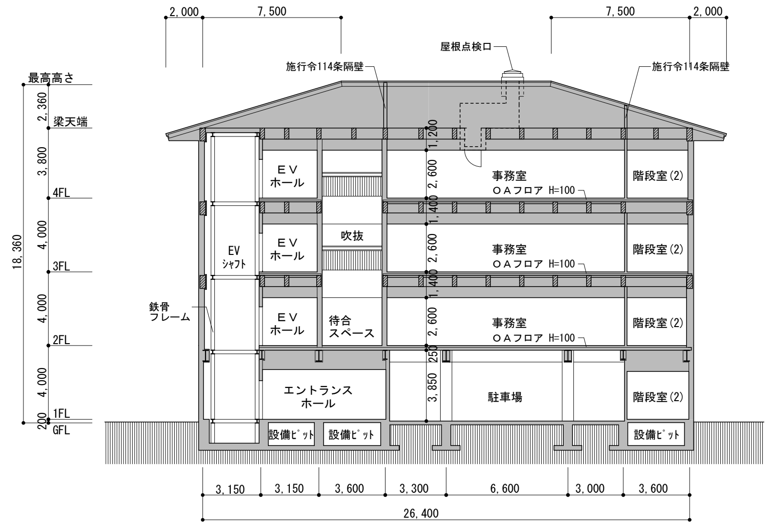
B-B' 断面図 1/200
