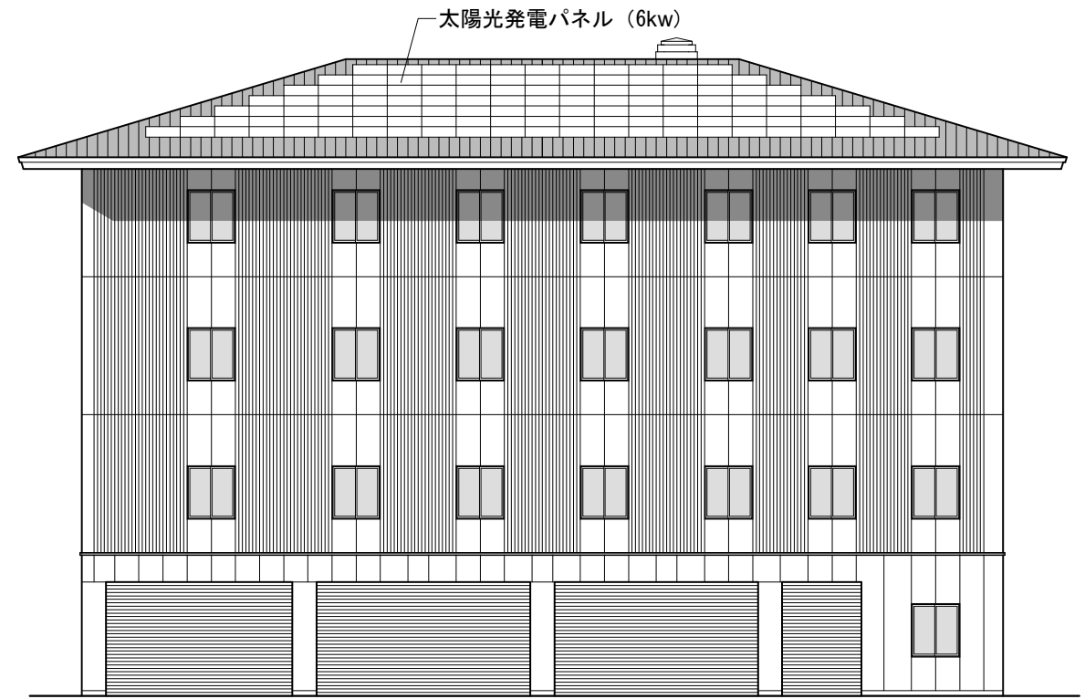
南側 立面図 1/200
