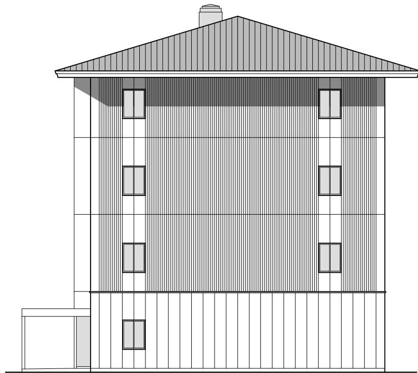
西側 立面図 1/200
