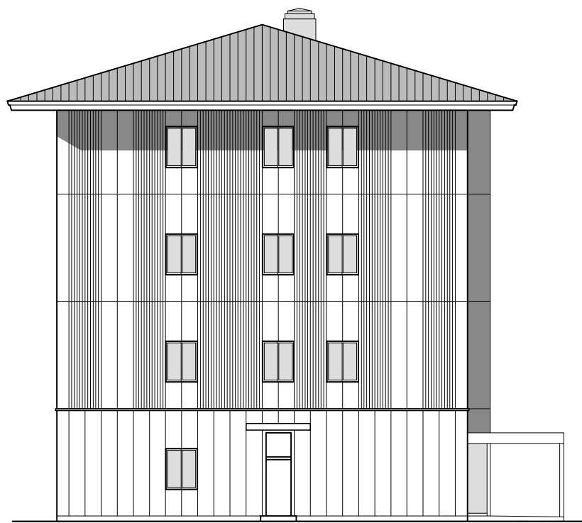
東側 立面図 1/200
