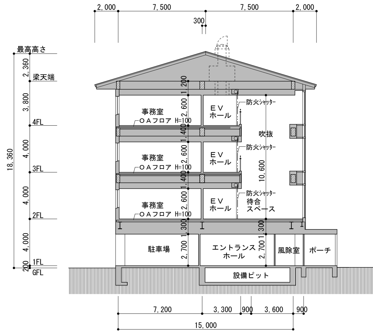
A-A' 断面図 1/200
