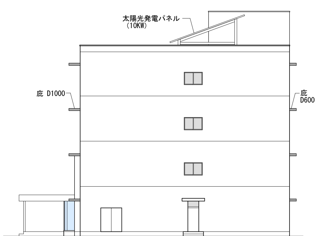
東側 立面図 1/200
