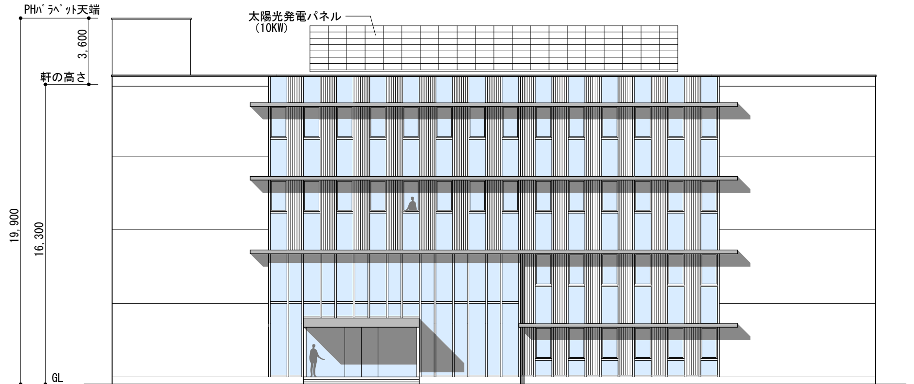
南側 立面図 1/200
