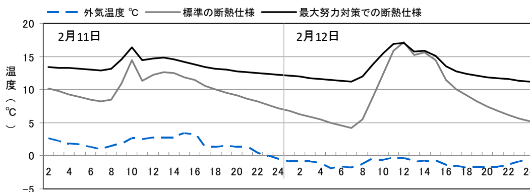
図 断熱仕様の違いによる床表面温度の時系列データ（仙台地域）
