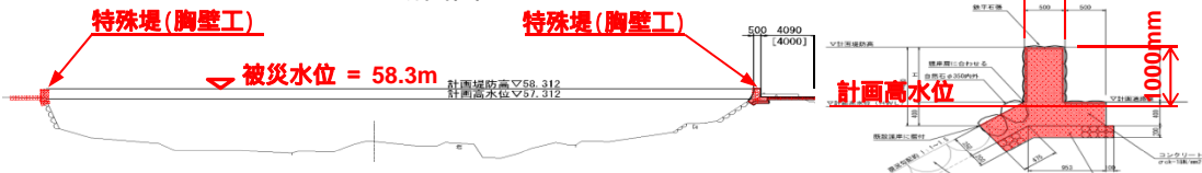
A-A'断面図
