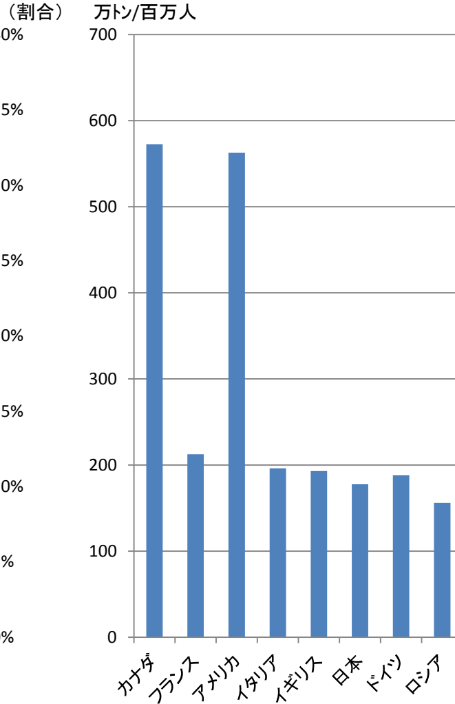
G8各国の人口当たり運輸部門CO 2 排出量 (2010年度)
