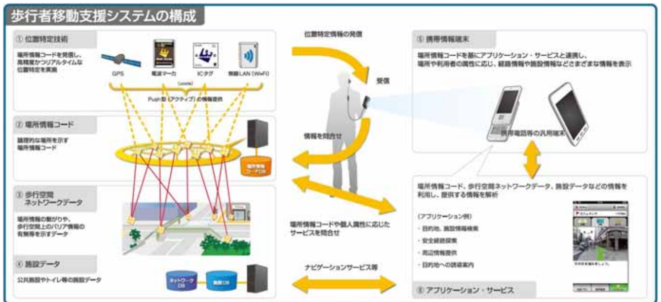
図 2-7 サービスに必要な技術要素
