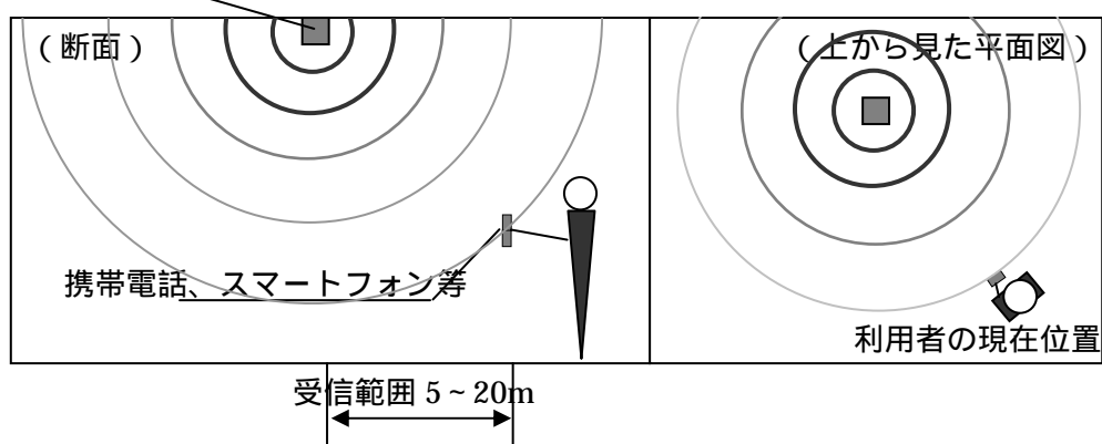
図 6-16 IMES の受信イメージ
