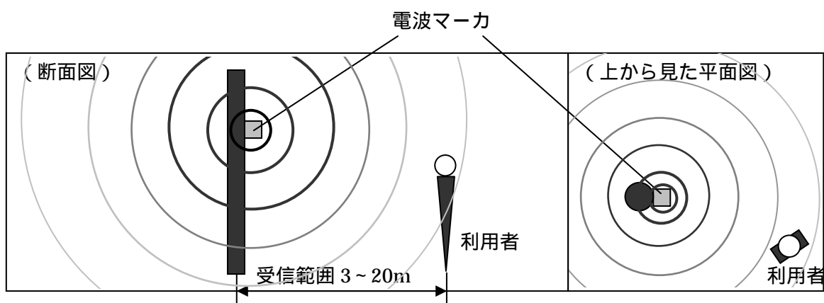
図 6-4 電波マーカの受信範囲イメージ
