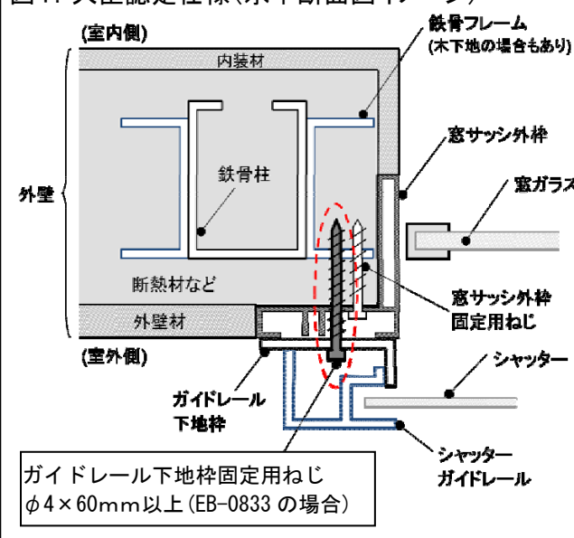
図1. 大臣認定仕様(水平断面図イメージ)
