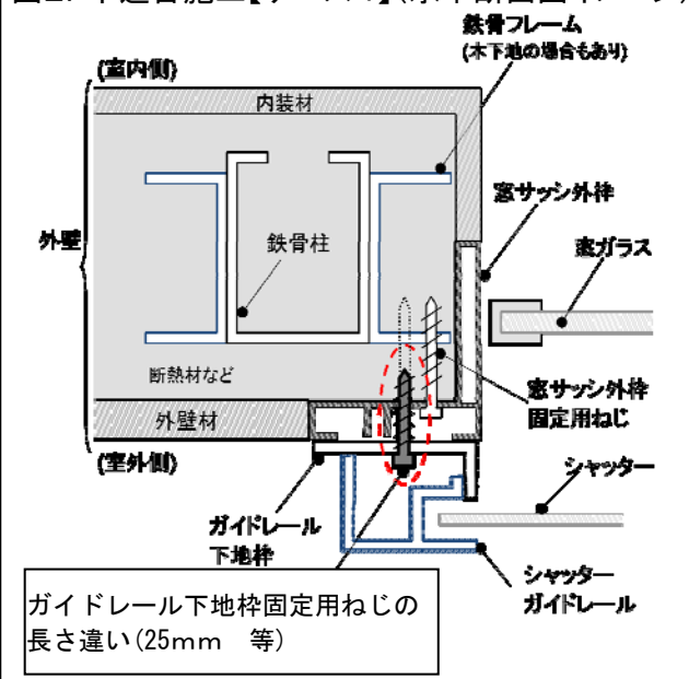
図2. 不適合施工【ケース1】(水平断面図イメージ)
