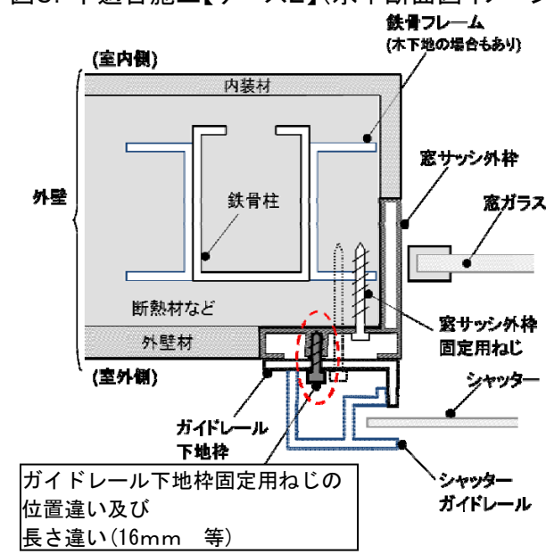
図3. 不適合施工【ケース2】(水平断面図イメージ)
