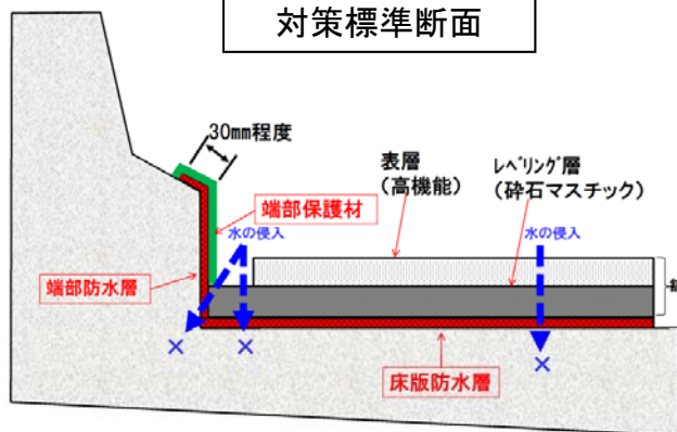
高性能床版防水の構造
