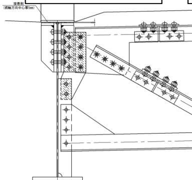
対策標準断面図
