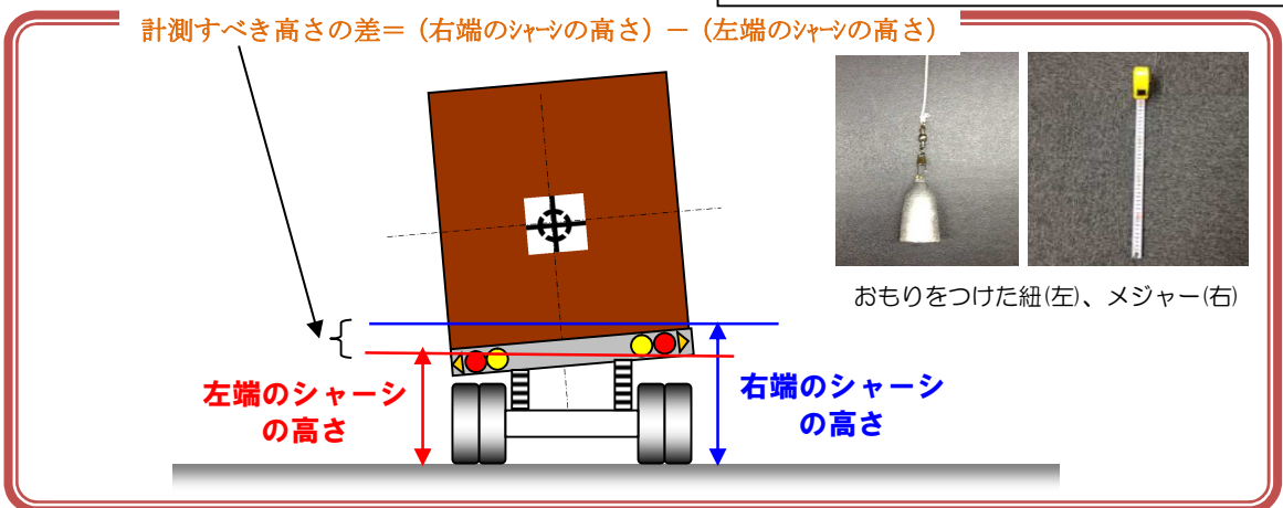
図5 トレーラー後部の左右の路面からの高さの差
