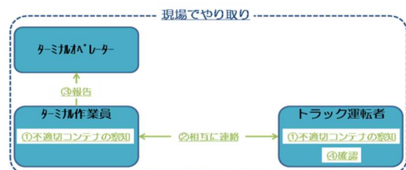
図15 偏荷重状態を察知した場合の連絡調整の経路
