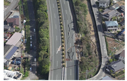
盛土法面の崩落(崩落延長約30~40m)
