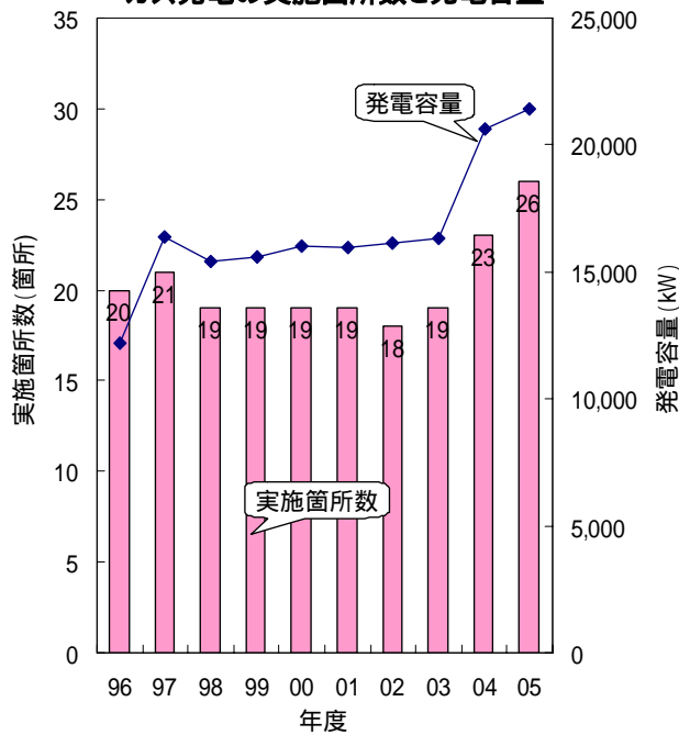
ガス発電の実施箇所数と発電容量
