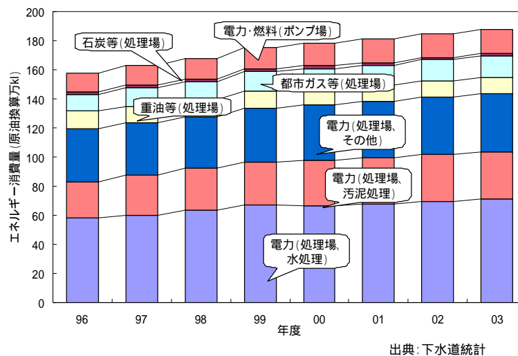
下水道施設のエネルギー消費量（一次エネルギー換算）
