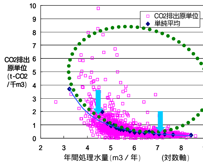
処理規模別の下水処理場の CO 2 排出原単位の平均値
