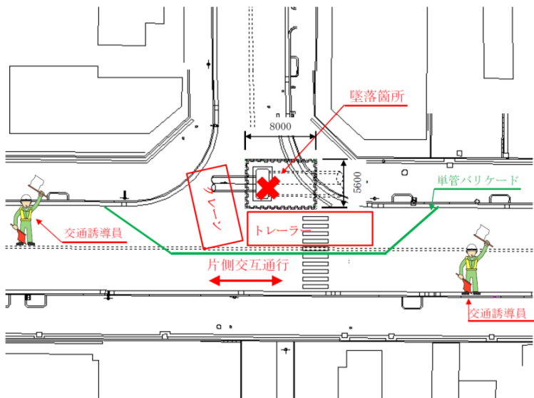
【平面図】
