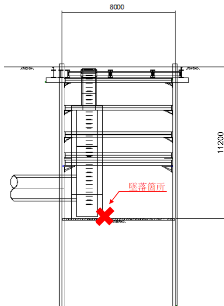
【断面図】
