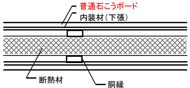
不適合 仕様 (水平断面図イメージ)
