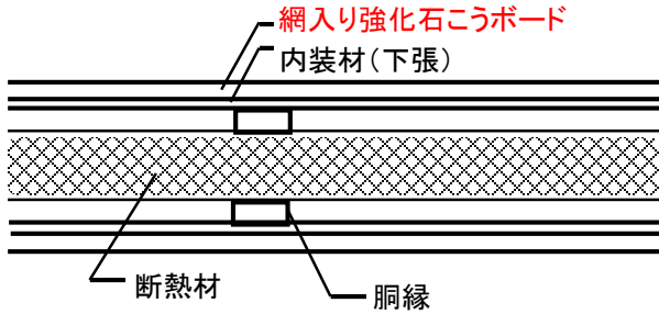
大臣認定 適合 仕様 (水平断面図イメージ)
