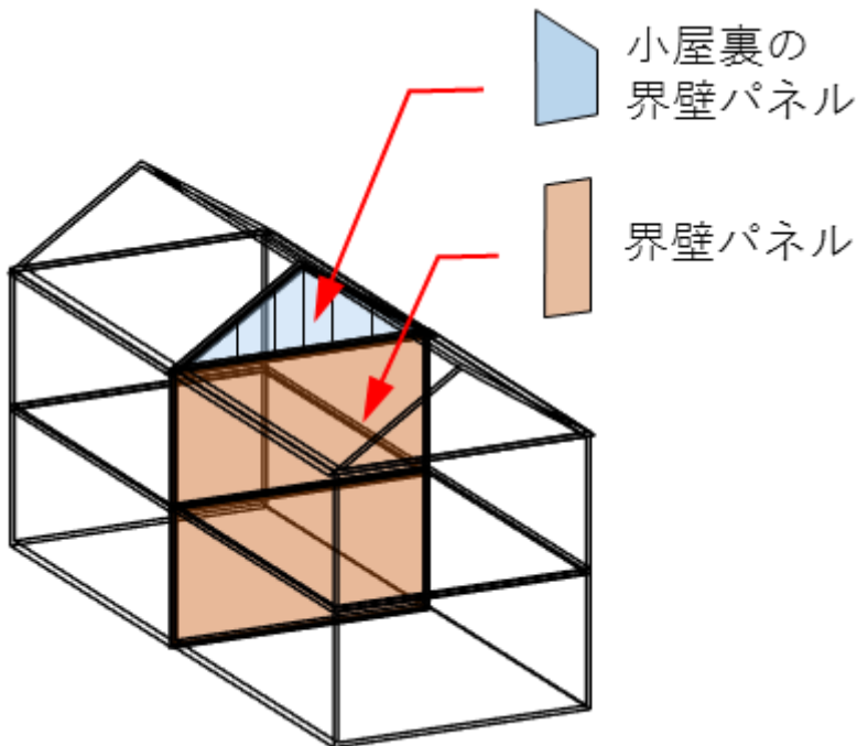
<小屋裏の界壁パネルの設置位置 イメージ>
