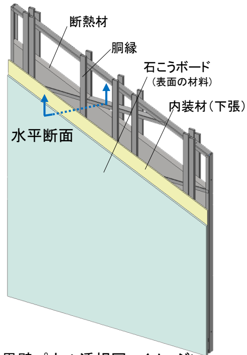
<小屋裏の界壁パネル透視図 イメージ>
