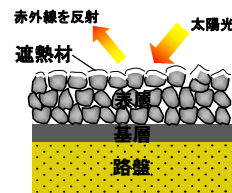
遮熱性舗装
