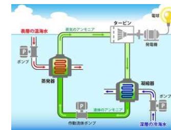
海洋温度差発電
