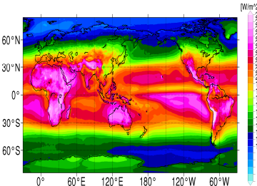
世界の年平均太陽放射量
