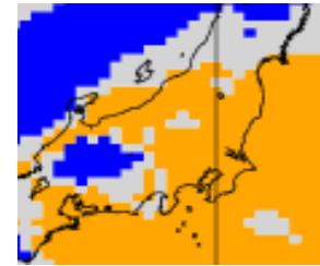
数値予報から算出した 天気分布図
