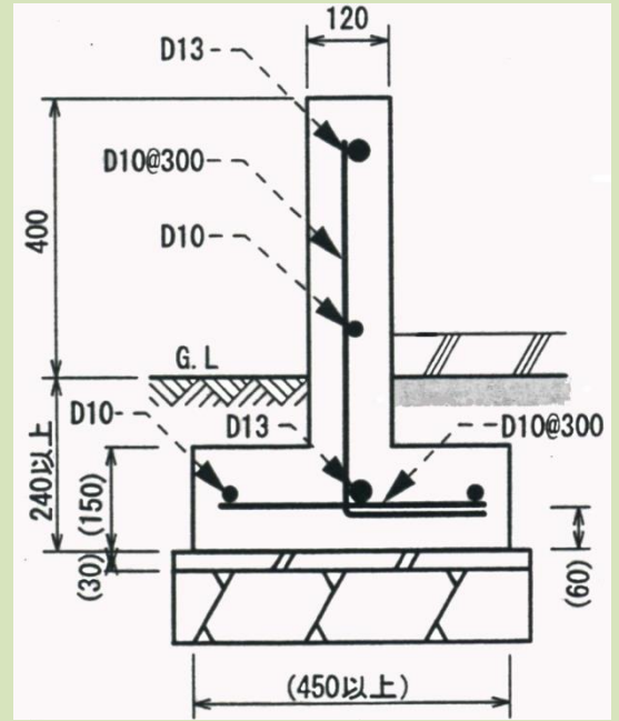
[住宅用基礎梁の形状例]
