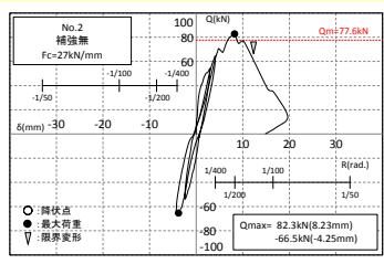
無補強梁の変形性状
