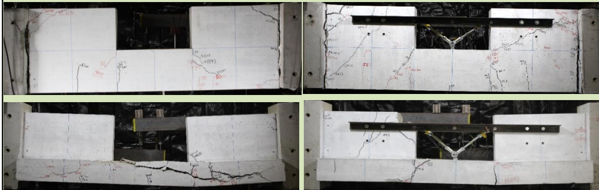
[平成26年度の人通口を有する梁実験の状況]
