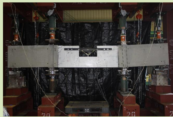
[構造実験手法と試験体破壊状況の一例]
