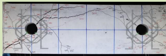
[平成26年度のスリーブを有する梁実験の状況]
