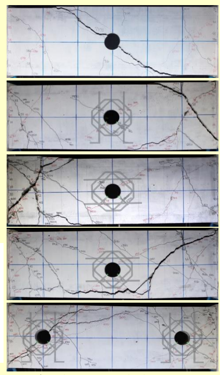
各試験体の破壊性状
