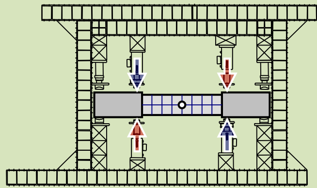
[構造実験手法と試験体破壊状況の一例]
