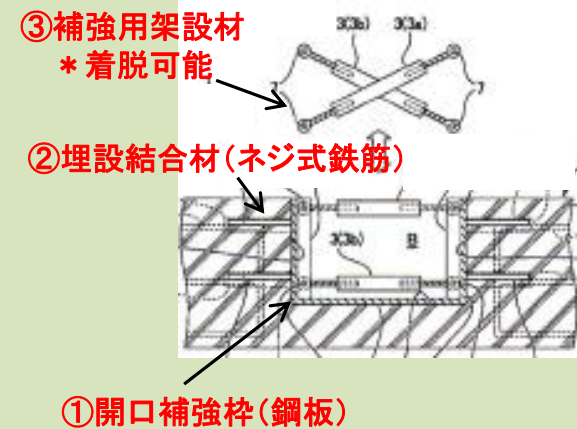
[点検補強システムの構成]
