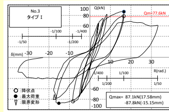
補強梁の変形性状
