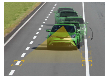
（車線逸脱抑制装置のイメージ）
