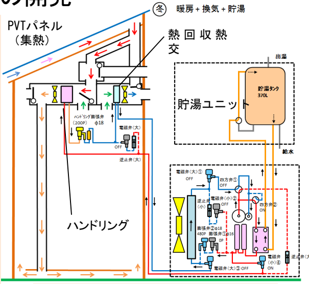
運転モード例 (暖房+換気+貯湯)
