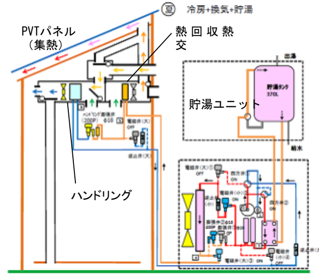
運転モード例 (冷房+換気+貯湯)
