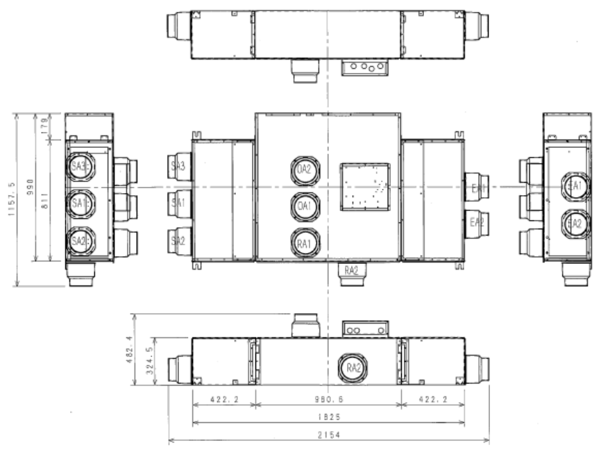
本開発の室内ハンドリングの外形図
