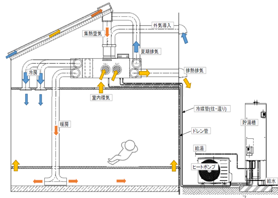
本開発システムの構成とダクト構成
