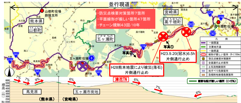
図5 国道218号の道路状況
