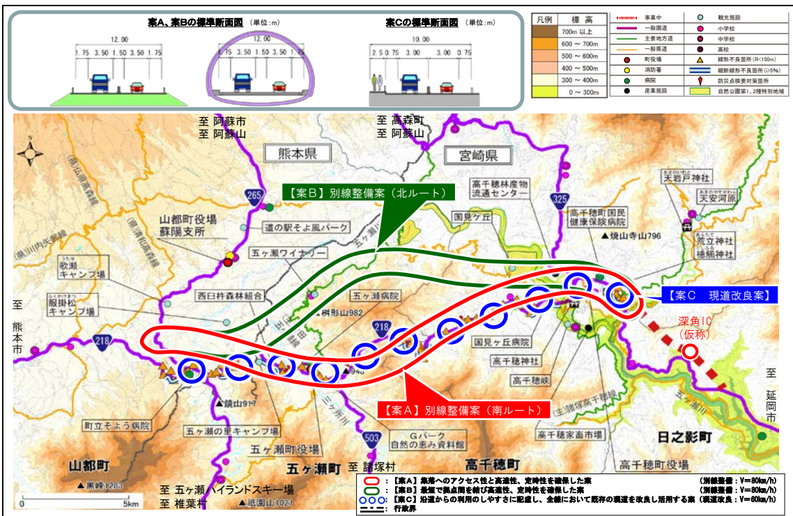
図6 蘇陽～高千穂における対策案検討
