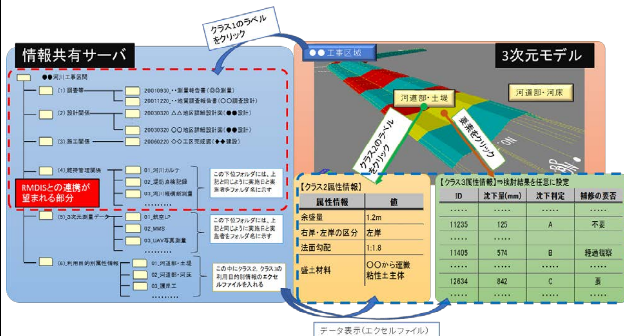
図 21 維持管理段階の河川 CIM モデルの例
