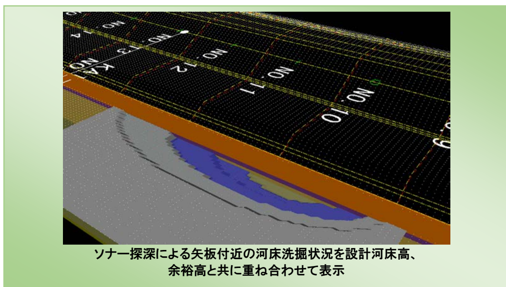
図 27 維持管理での活用イメージ（適切な矢板護岸管理）
