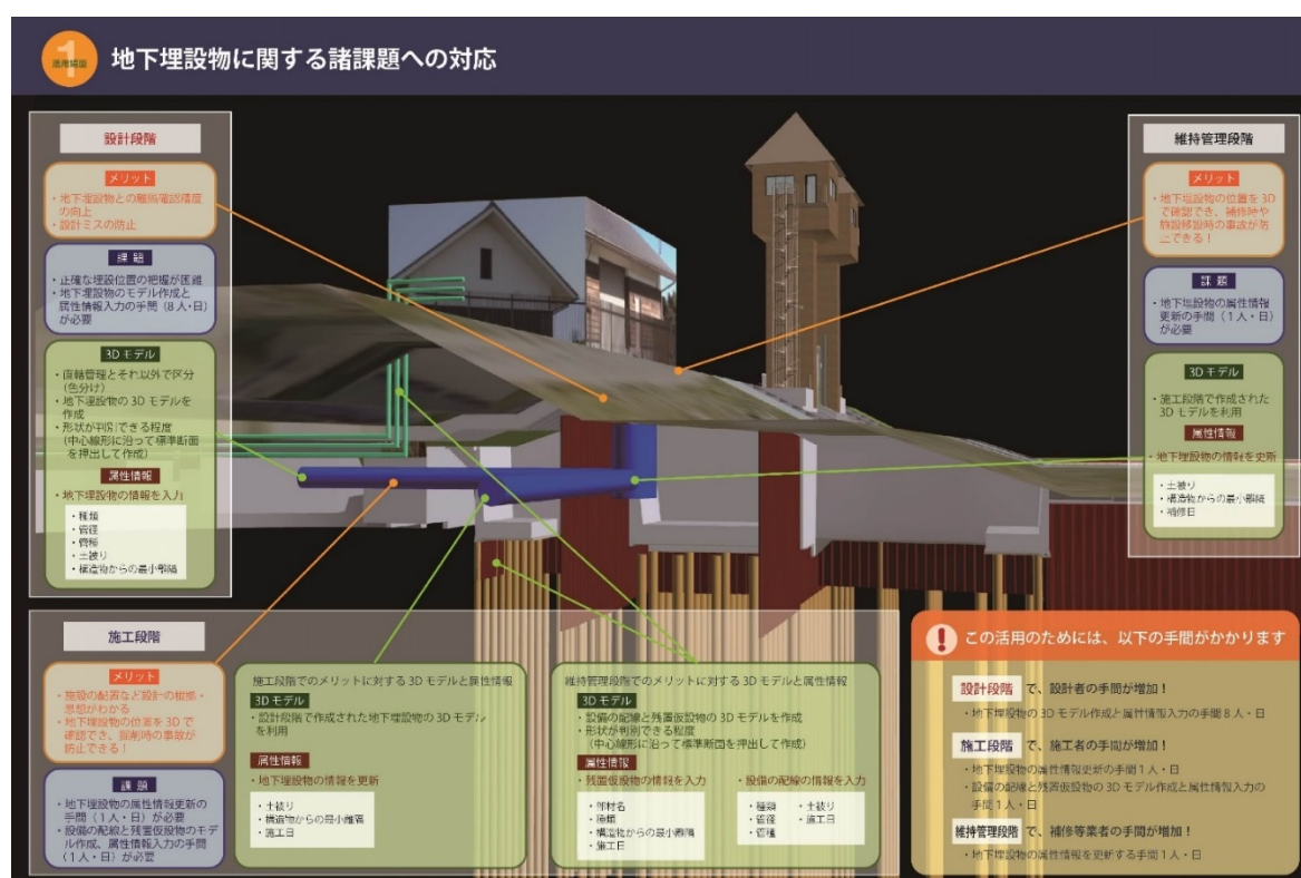
図 24 維持管理での活用イメージ（地下埋設物管理）
