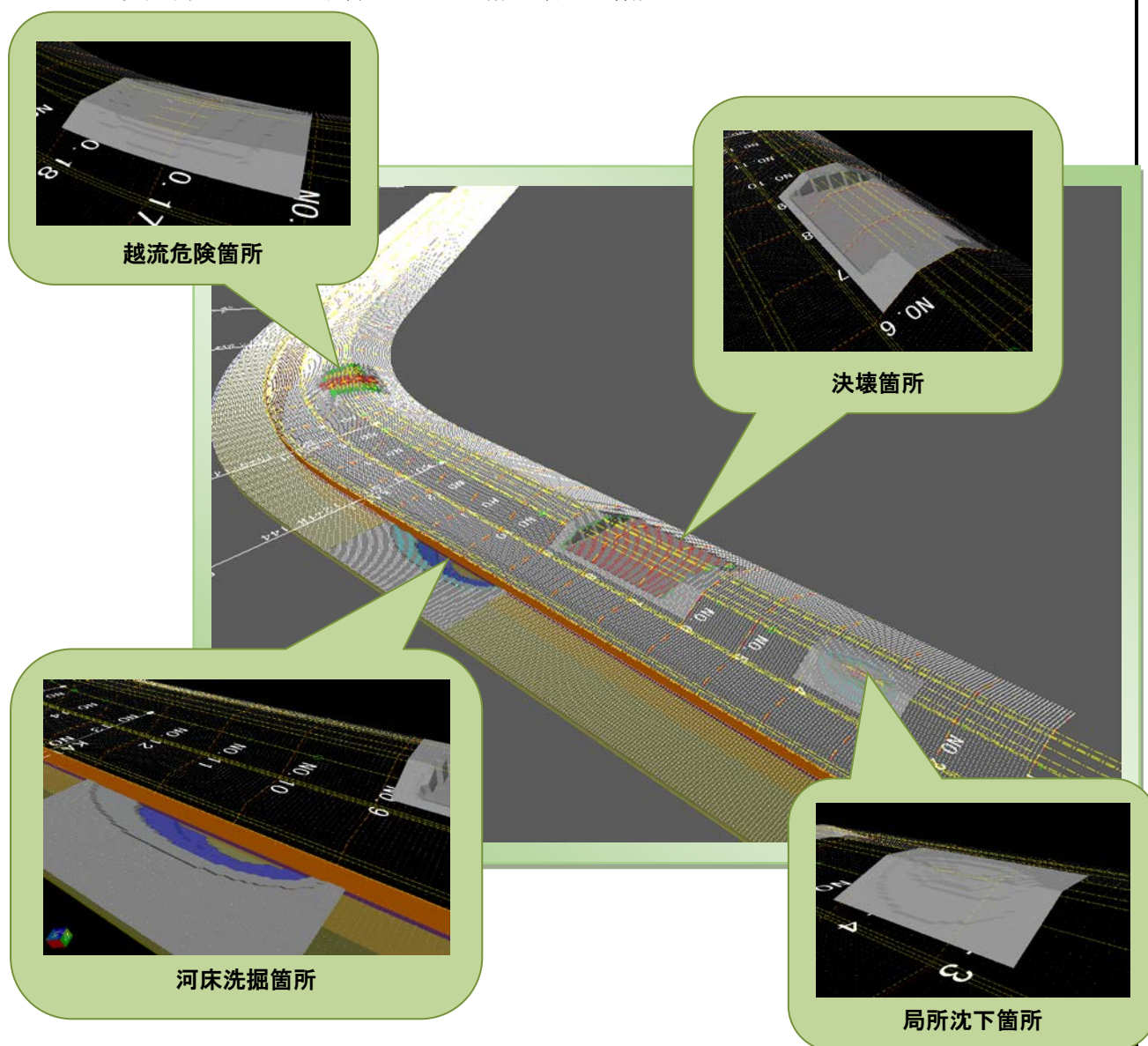
図 26 維持管理での活用イメージ（河道管理の高度化）
