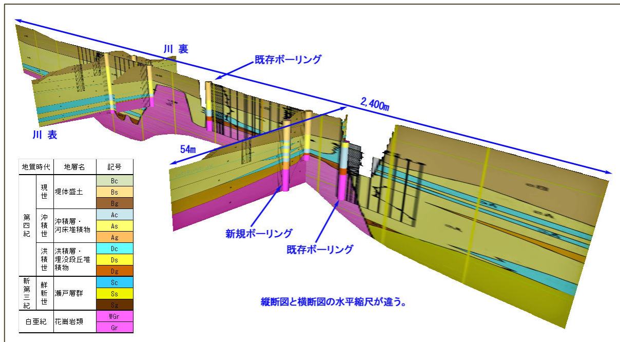
図 7 河川堤防(堤防地質縦断面図、横断面図、ボーリング)の3次元表示例
