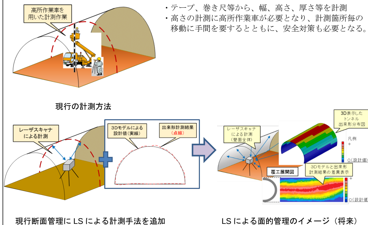
図 20 トンネルでの新たな手法による出来形管理
