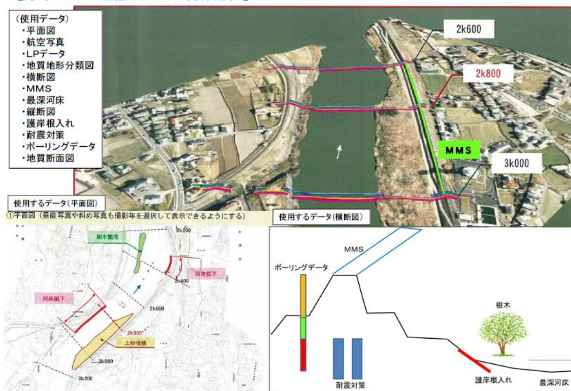
図 29 基本フレームのイメージと河川 CIM の整備イメージ(最終形)
