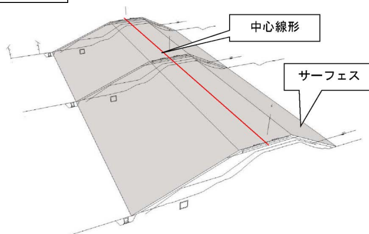
図 11 骨格構造モデル（スケルトンモデル）とサーフェスモデルの例（堤防）
