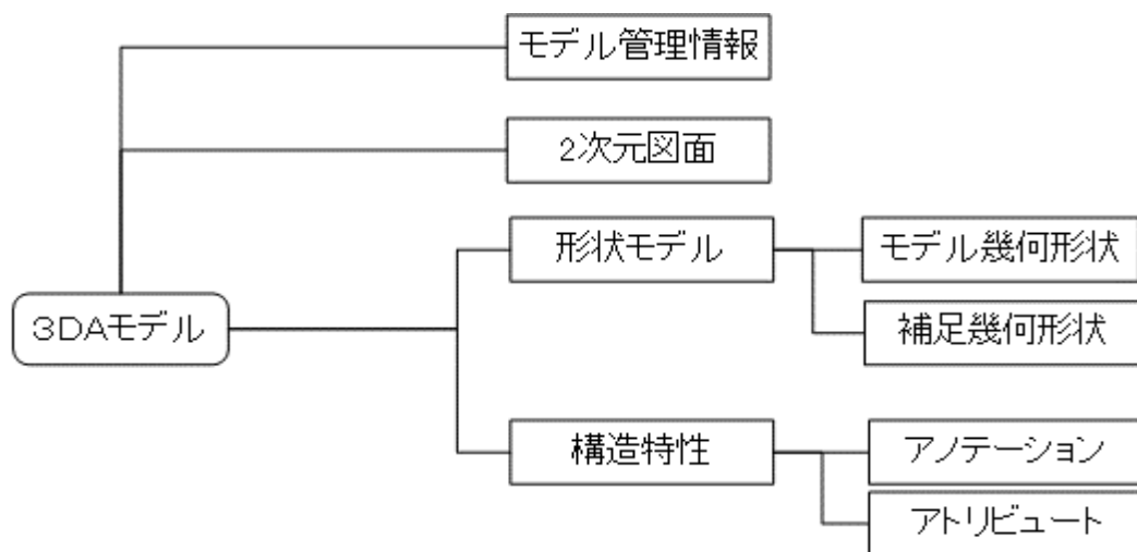
図 4-1 3DA モデルの情報構成
