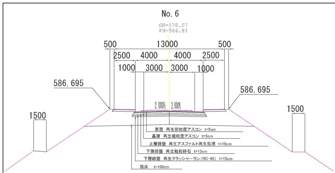
図 4-8 横断面図の例
