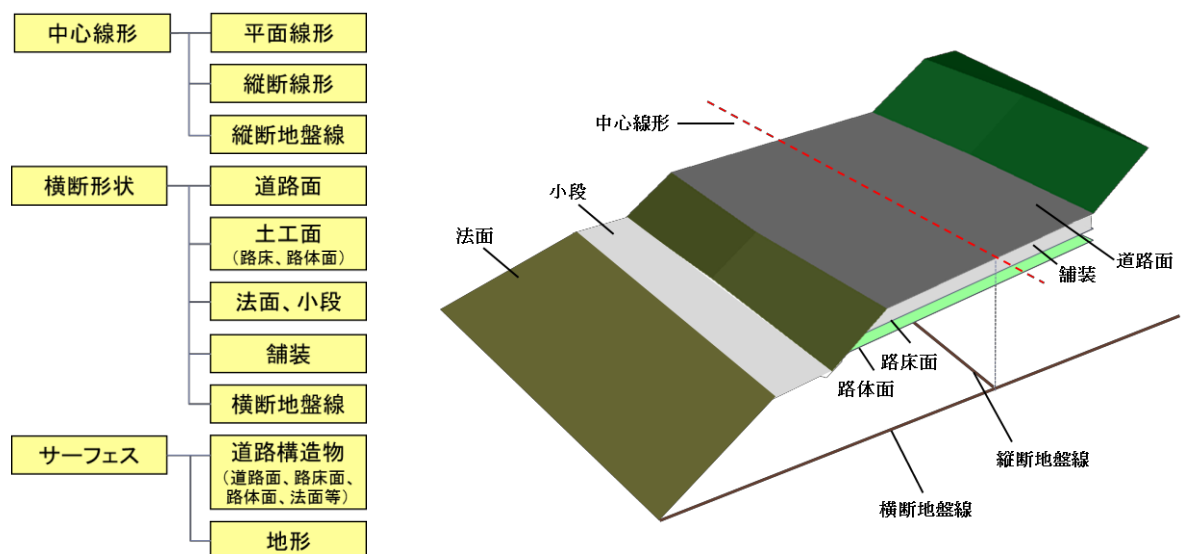
図 4-2 道路土工の形状モデルの構成要素イメージ図
