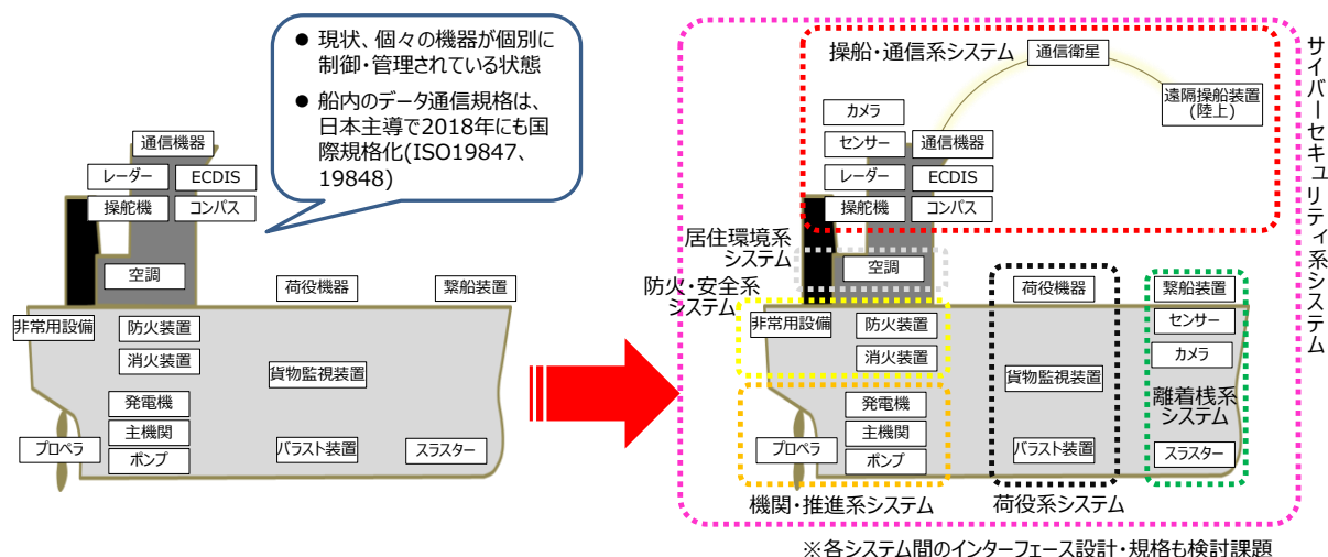
図 22 システム化・モジュール化のイメージ
