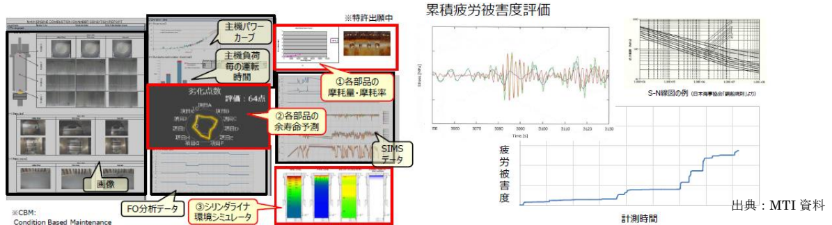
図 17 機関の予防保全・船体モニタリングのイメージ
