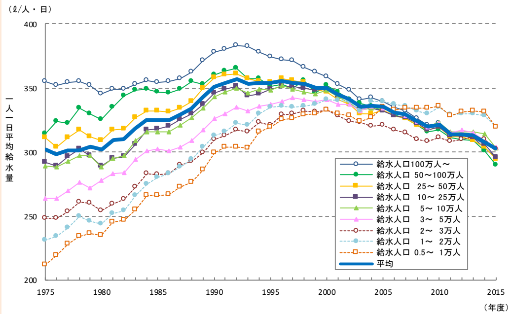
図2-2-5 上水道事業の月別一日平均給水量
