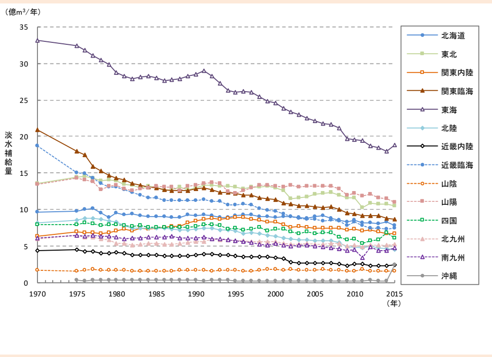
図 2-3-3 地域別工業用水回収率の推移
