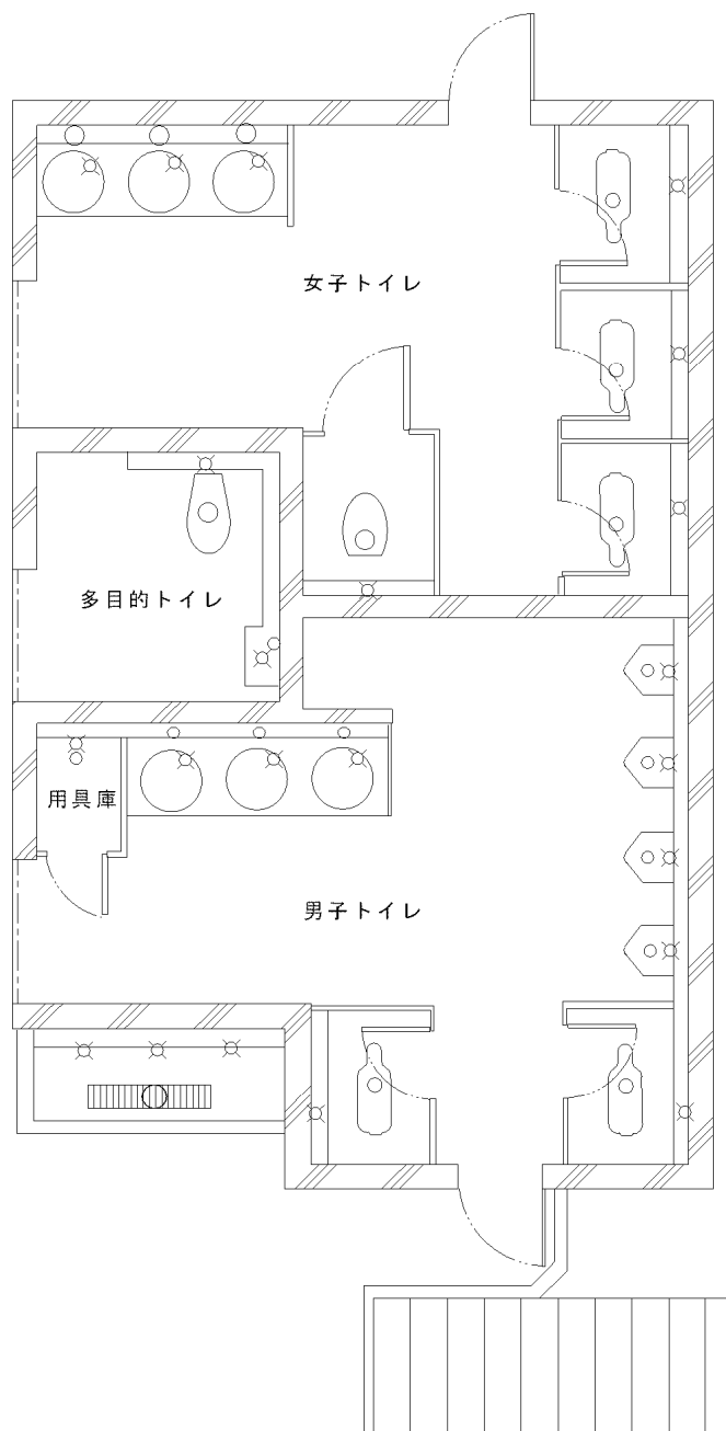
管理事務所前便所 1階平面図
