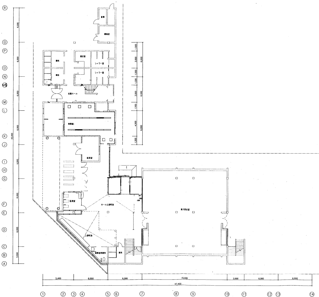
1階平面図
