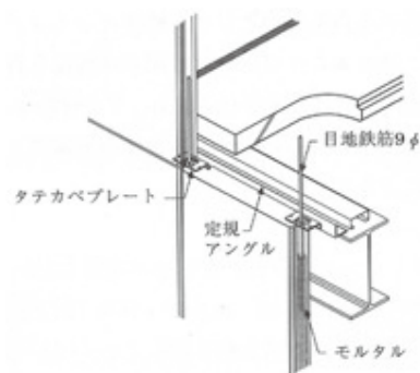
ALCパネル縦壁挿入筋工法の施工納まり参考図
