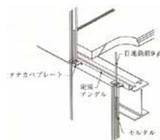
[図02] ALCパネル縦壁挿入筋工法の施工納まり参考図
