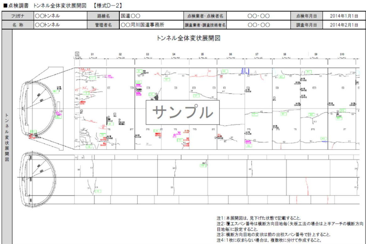
図 2-7 トンネル変状展開図の例
