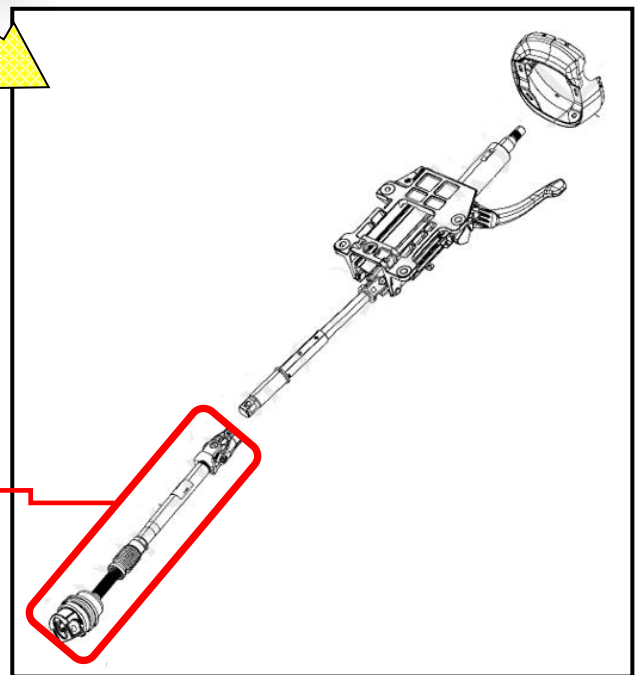
ステアリングコラムシャフトアッセンブリ
