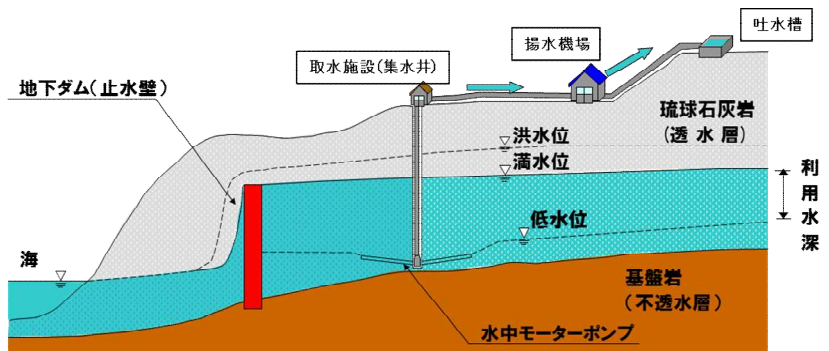
地下ダム 概要図
