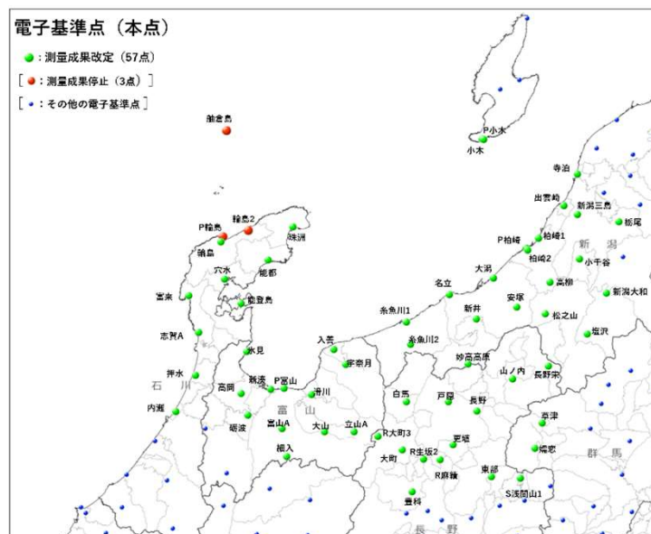
電子基準点の位置情報改定状況（2月7日公表）
