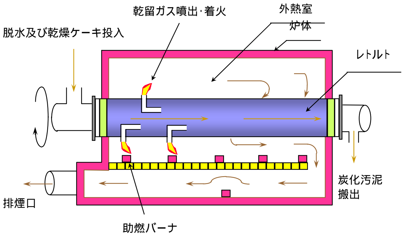
汚泥炭化システム
