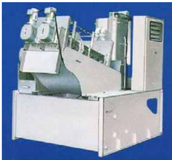
多重板外押型スクリーブレス脱水機
