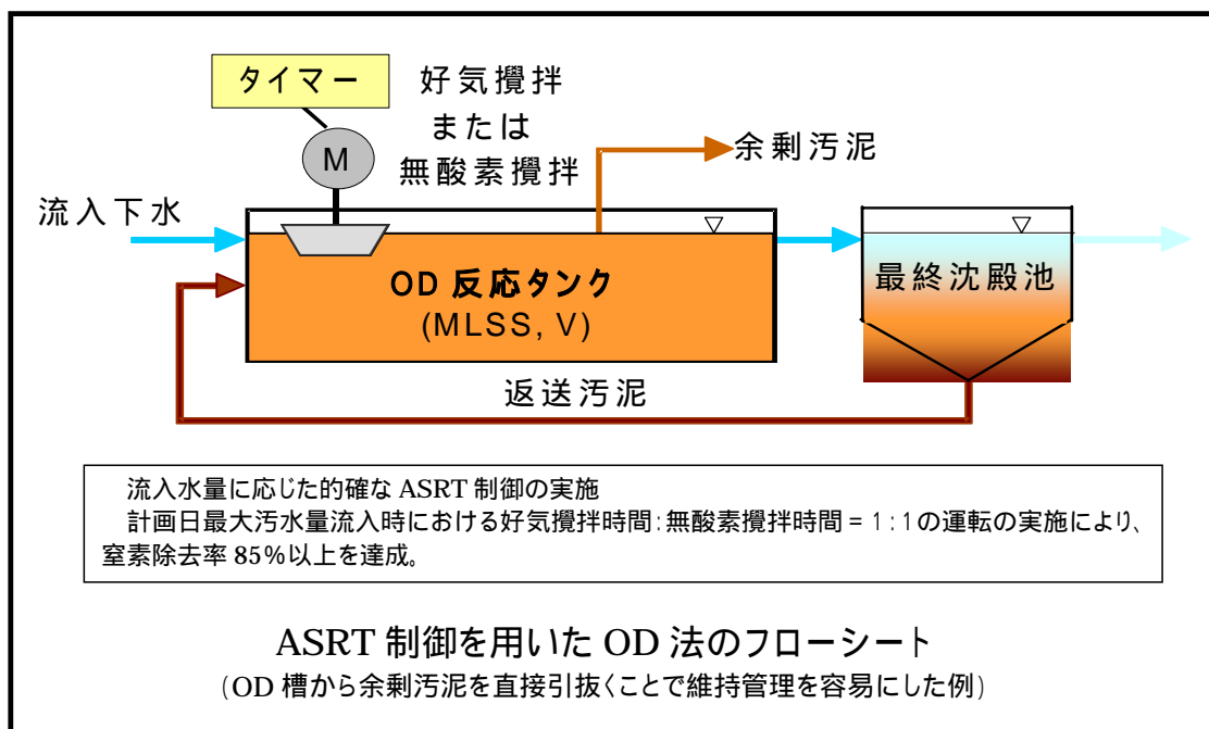
高度処理対応型 OD 法
