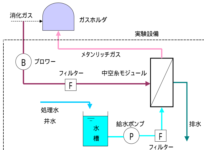
下水汚泥消化ガスの活用
