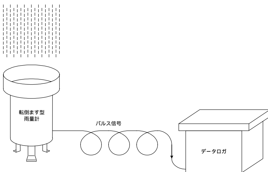
図 3-1 転倒まず型雨量計の構成例
