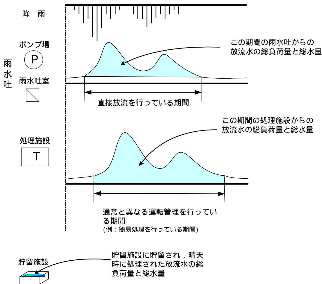
図 2-2 雨水の影響が大きい時の放流負荷量と放流量
