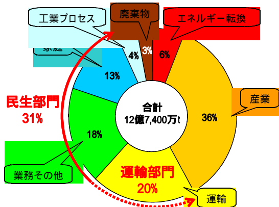
我が国の部門別の二酸化炭素排出量(2006年度)
