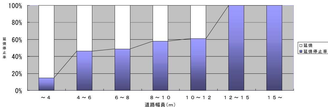
道路幅員別の延焼防止率 (阪神・淡路大震災における神戸市長田区の事例)
