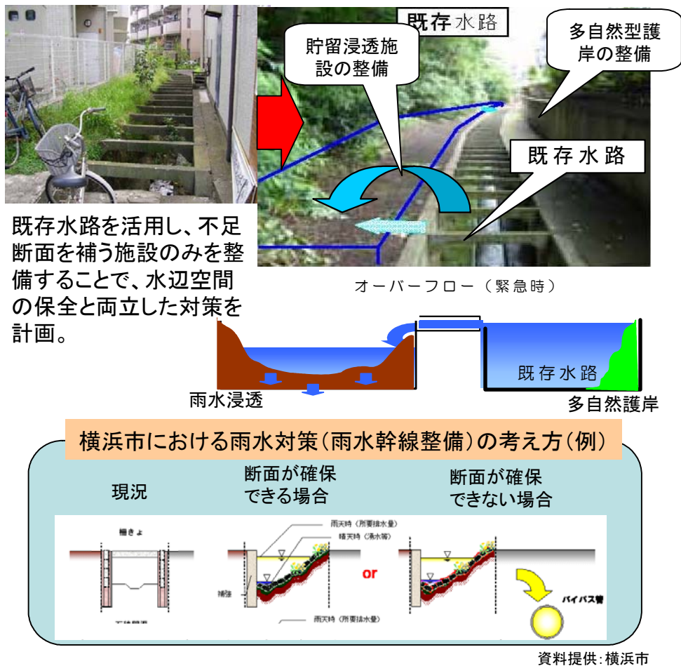
図—1 4 雨水対策における水面の確保（横浜市）
