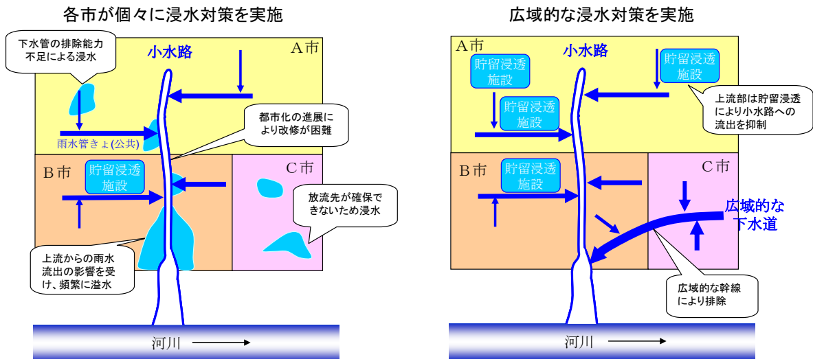
図－１７ 上下流一体に捉えた広域的な浸水対策
