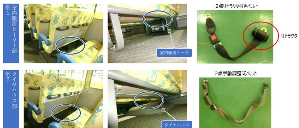
幼児用の2点式リトラクタ付座席ベルトを備えられない場所の例
