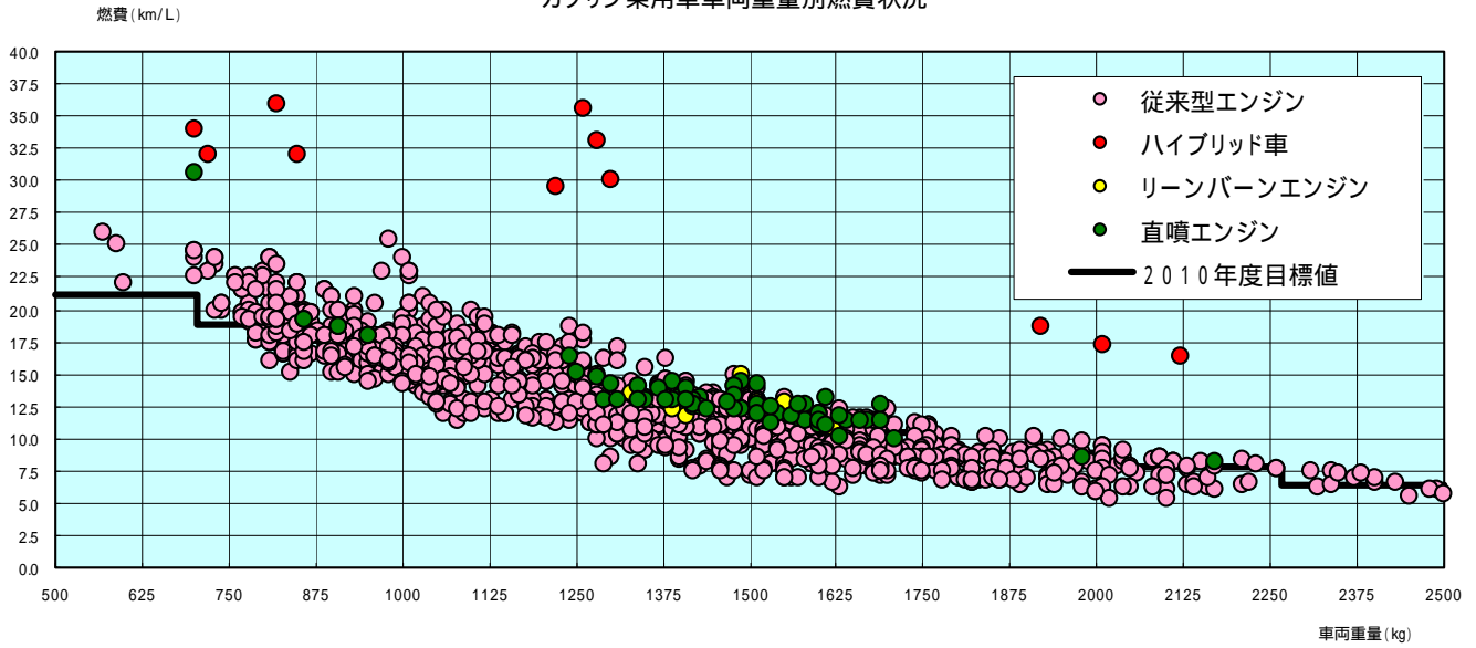
ガソリン乗用車車両重量別燃費状況
