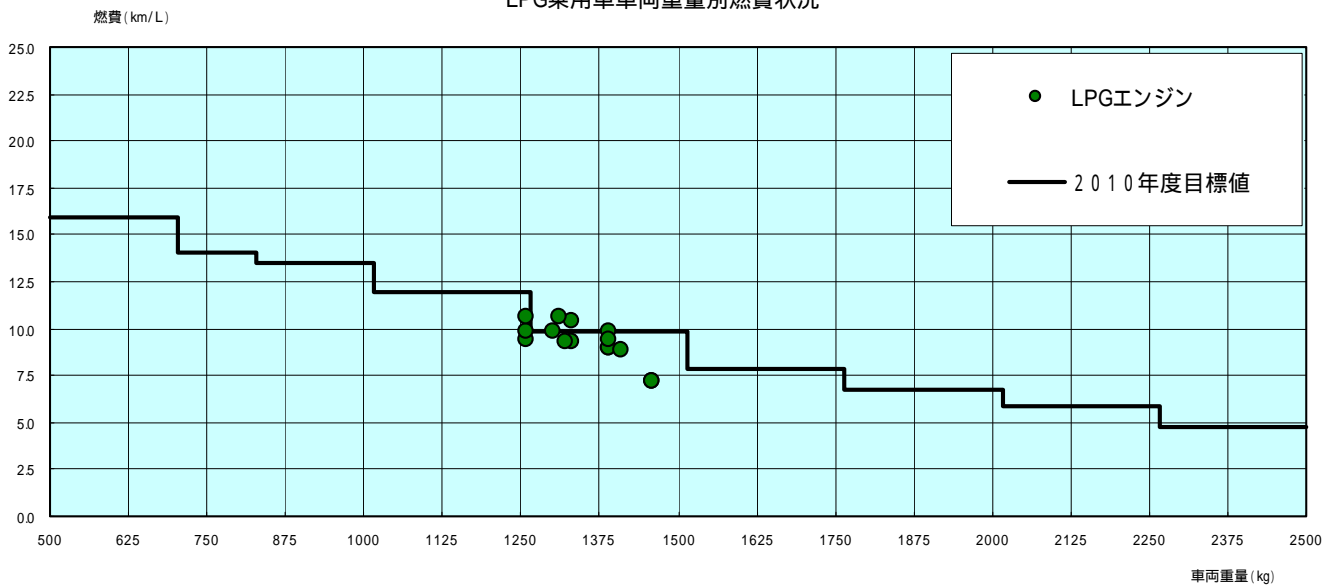
LPG乗用車車両重量別燃費状況
