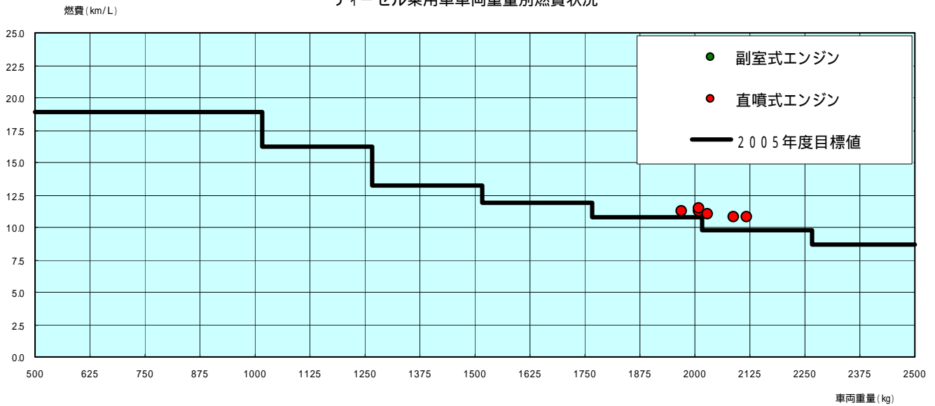
ディーゼル乗用車車両重量別燃費状況
