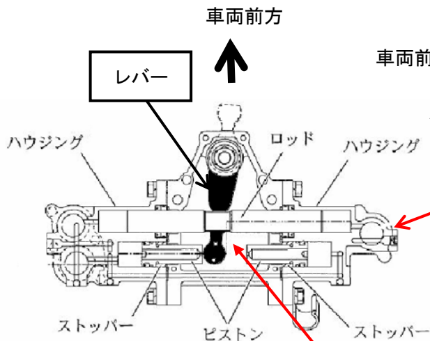
変速ユニットを上面から見た図
