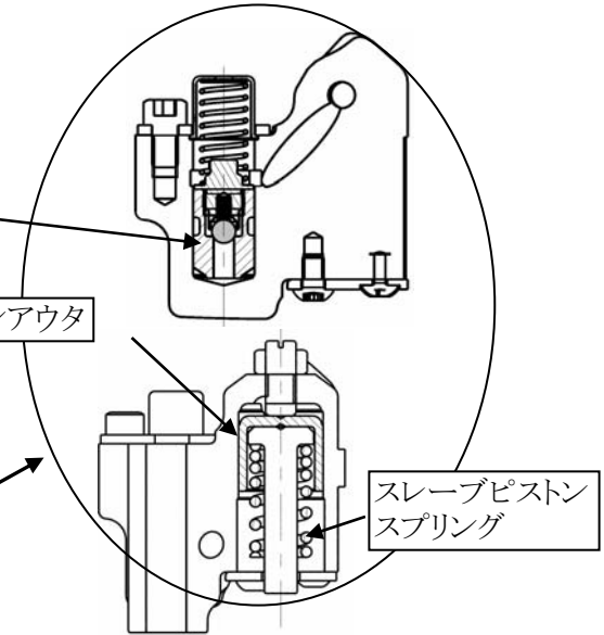
コントロールバルブ
