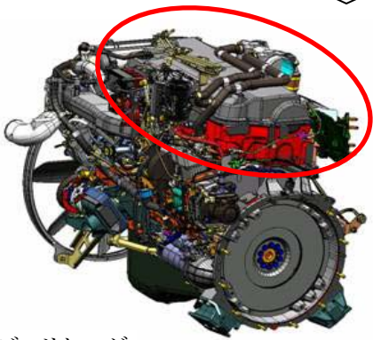
エンジンリターダ 上面視
