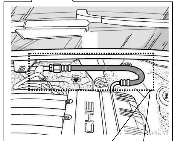
燃料ホース
