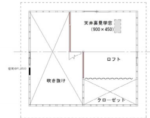
2 階平面図
