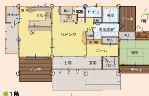
<展示住宅・生活体験施設の平面図>
