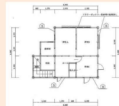
2階平面図
